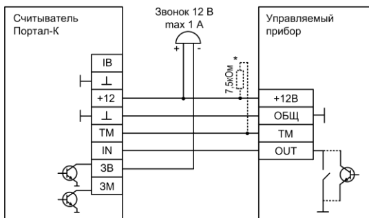
* - при неустойчивом считывании данных с Портала-К необходимо подключить резистор 7,5 Ом между контактами «TM» и «+12В» управляемого прибора.
